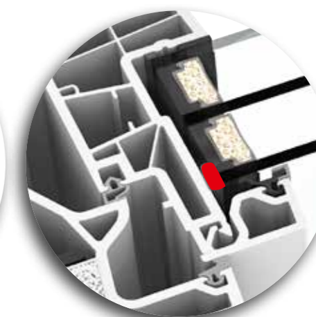
Oszklenie I-tec
