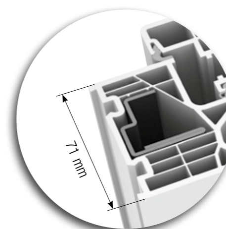
Głębokość profilu
